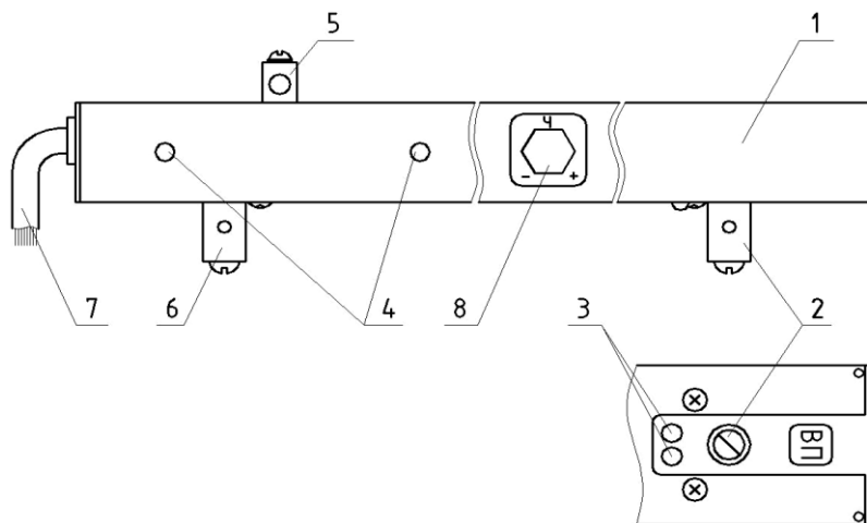
Рисунок 1.3 Конструкция ПРМ.
